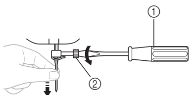
① Отвертка ② Винт иглодержателя
