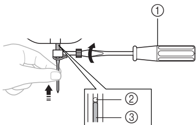
① Отвертка ② Стопор иглы ③ Игла
